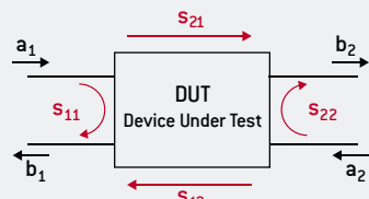
Figure 2: S parameters
