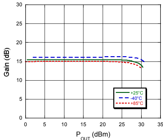
P1dB
