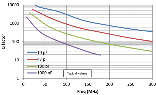
Q factor: 3838/S58E
