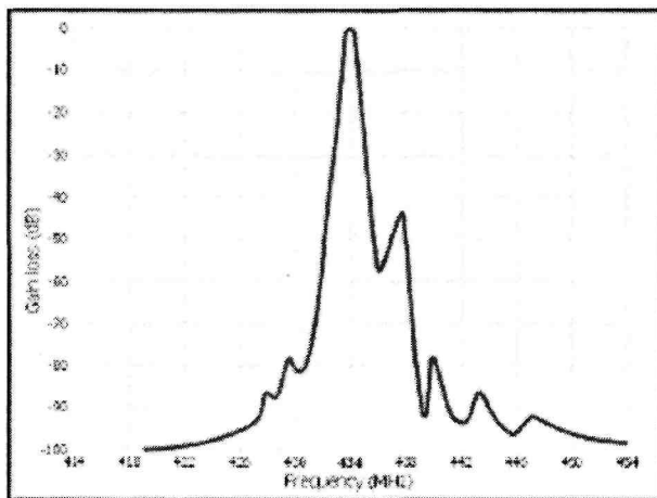
Fig.4 Grafico Frequenza-Selettività
